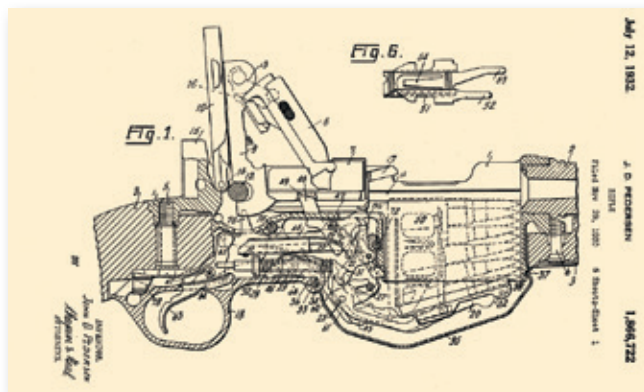
Contrairement au Garand, le bloc détente est solidaire des mécanismes de blocage et d'éjection du clip, ainsi que de l'élevateur de cartouche. Les pièces du mécanisme sont en alliage coulé, de type Zamac.
